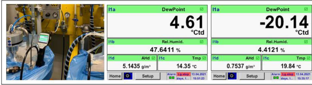
Şekil 3.2. Nem ölçümü
